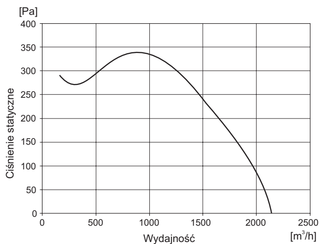
KEF-4-200/74-055
