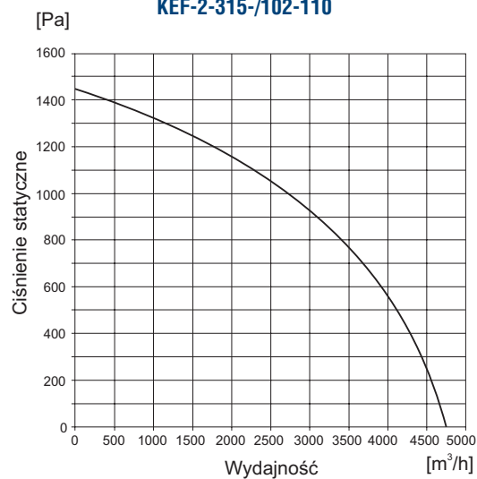
KEF-2-315-/102-110
