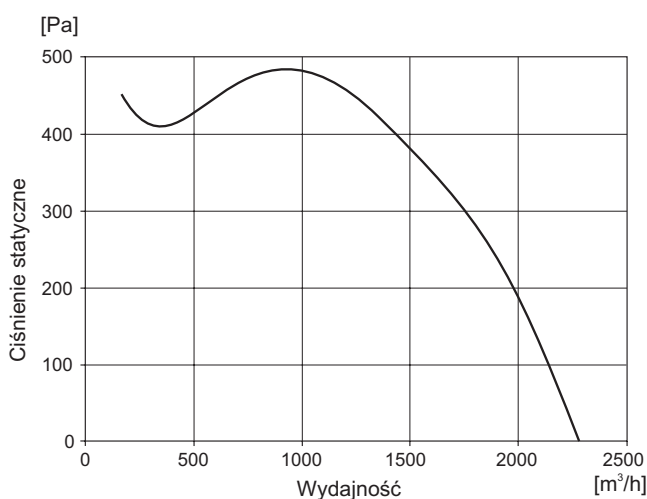
KEF-4-250/114-110
